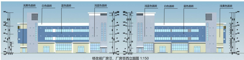
修改前厂房Ⅱ、厂房Ⅲ西立面图 1:150
