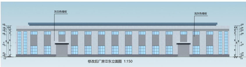
修改后厂房Ⅱ东立面图 1:150
