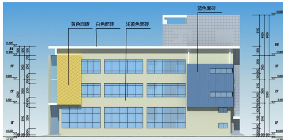
修改前厂房Ⅱ、厂房Ⅲ侧面图1:150
