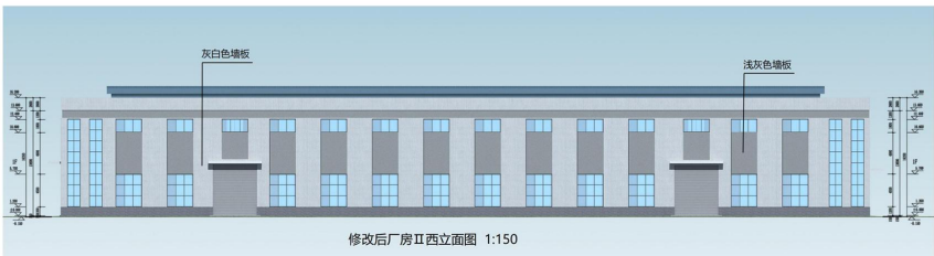
修改后厂房Ⅱ西立面图 1:150
