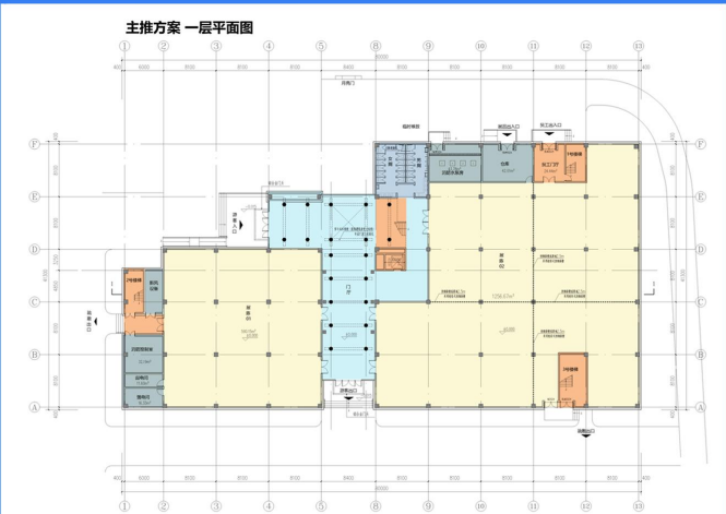
一层平面图 本层建筑面积：2790.76㎡，本层计容面积：5581.52㎡，本栋楼建筑面积：4985.55㎡，
