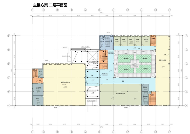
二层平面图 本层建筑面积：2194.79㎡，本层计容面积：4389.58㎡
