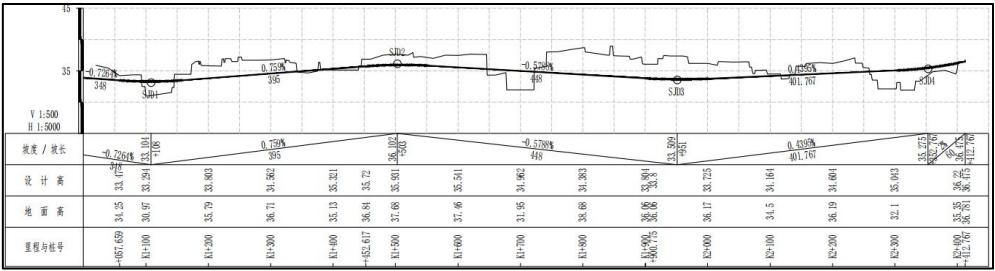
图 2.3-2 纵断面设计图
