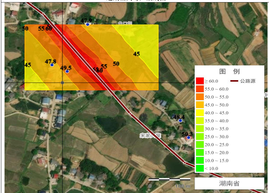
远期夜间等声级线图
