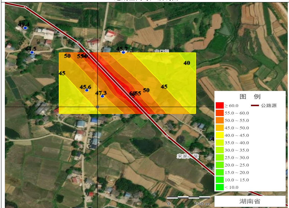
近期夜间等声级线图
