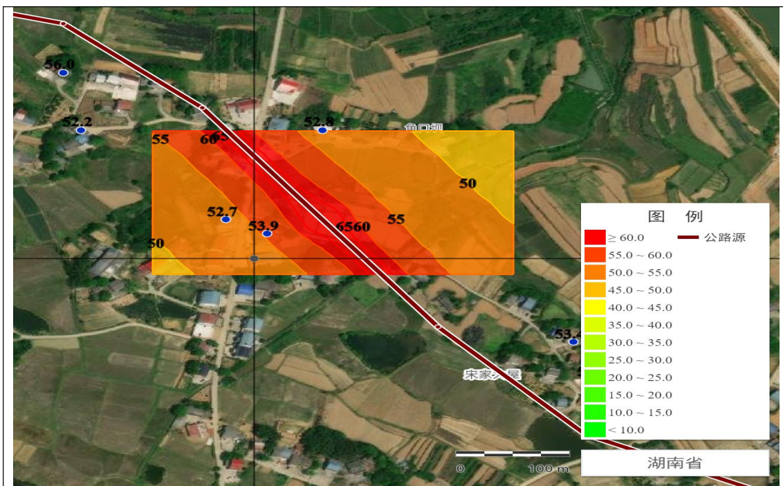
中期昼间等声级线图
