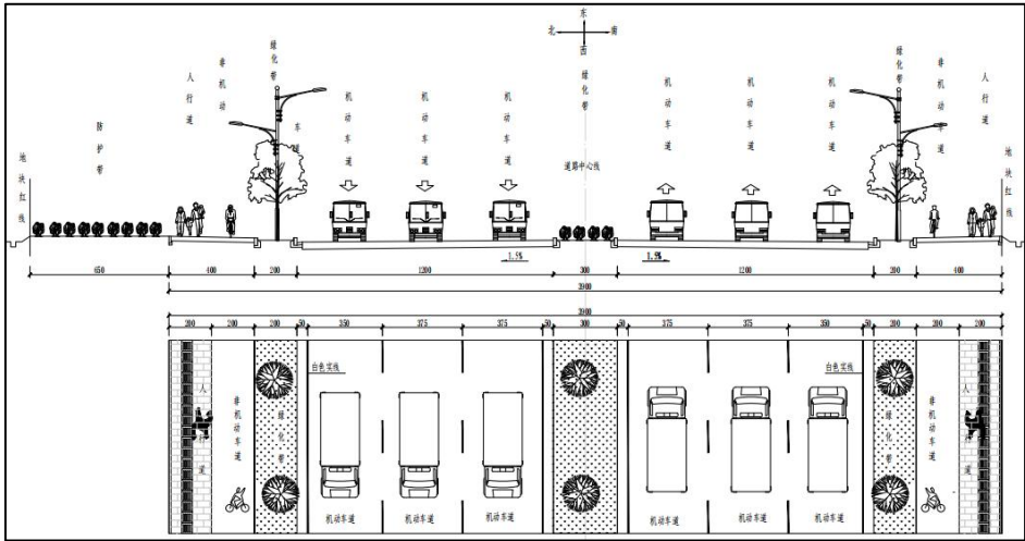
图 2.3-4 交叉口拓宽段横断面图
