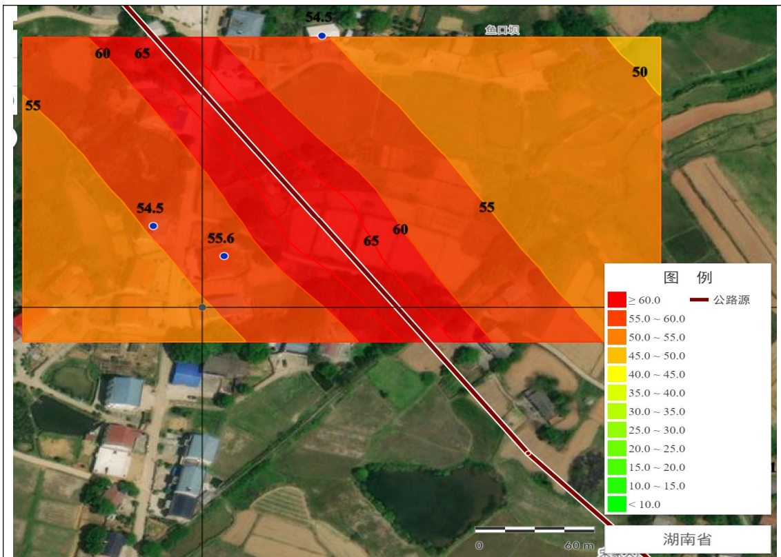
远期昼间等声级线图
