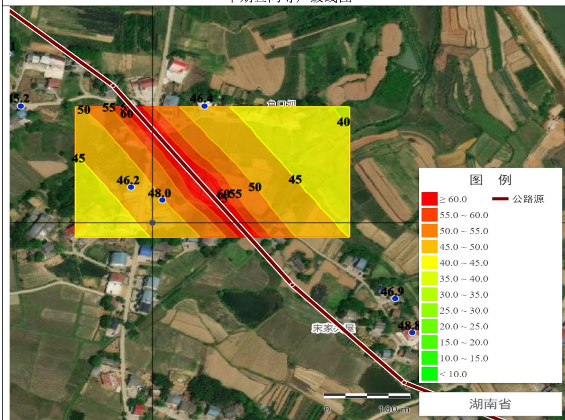
中期夜间等声级线图
