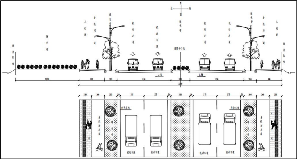
图 2.3-3 道路标准横断面图
