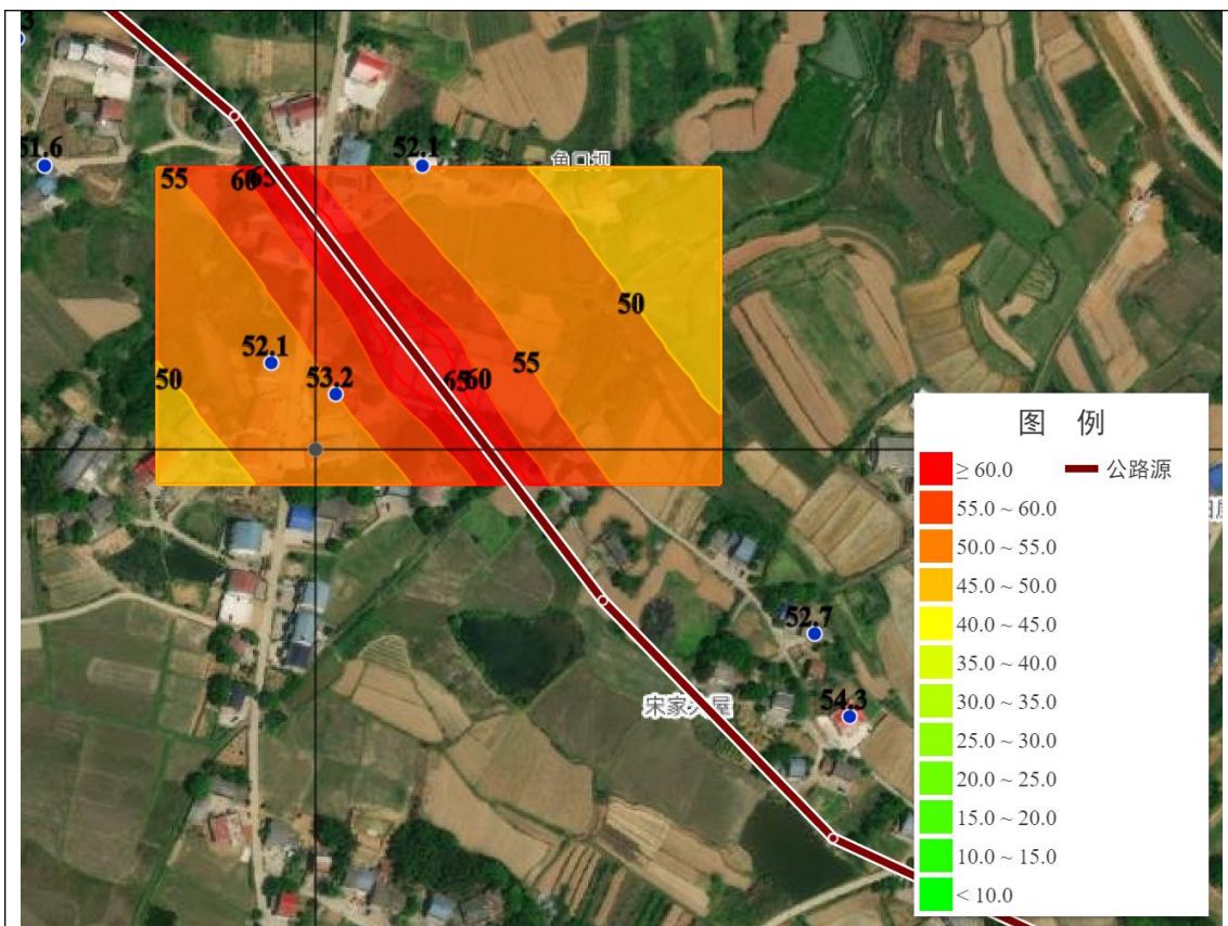
近期昼间等声级线图
