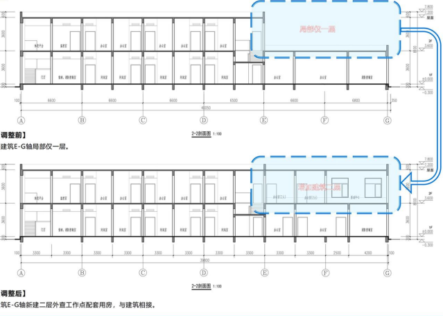
调整前后建筑方案对比
