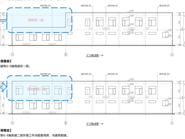
调整前后建筑方案对比
