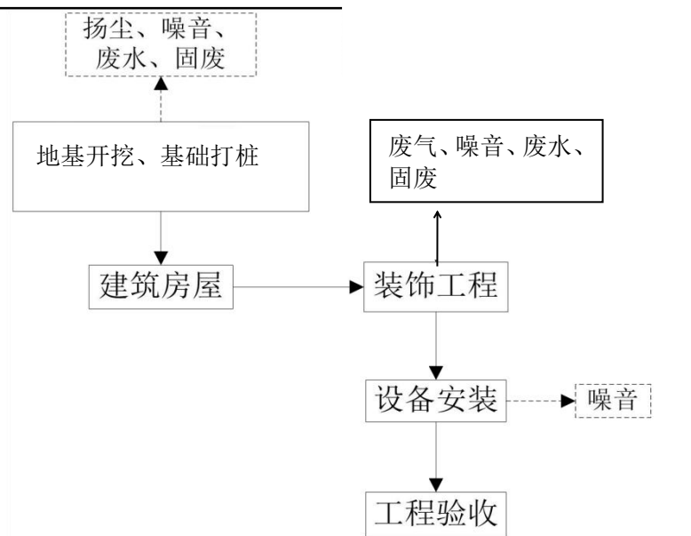
图 2-2 施工期工艺流程及产污位置图
